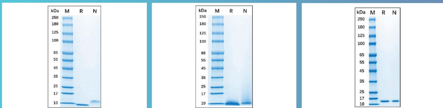
还原性(R)和非还原性(N)条件下进行SDS-PAGE实验的结果
